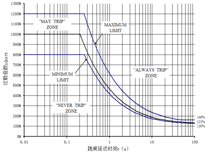
图1 跳闸保护曲线
