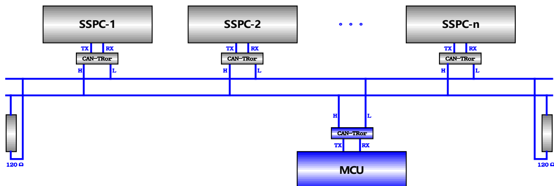
图8 模块组网拓扑结构
