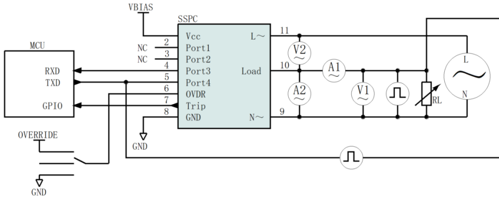
图9 SCI 型模块测试电路
