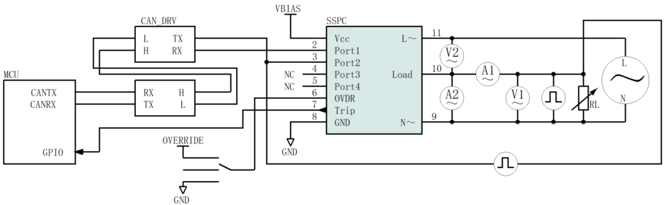
图11 CAN 型模块测试电路
