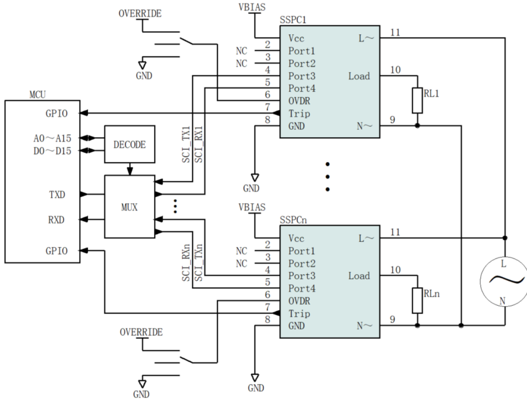
图4 多 SCI 接口模块交联
