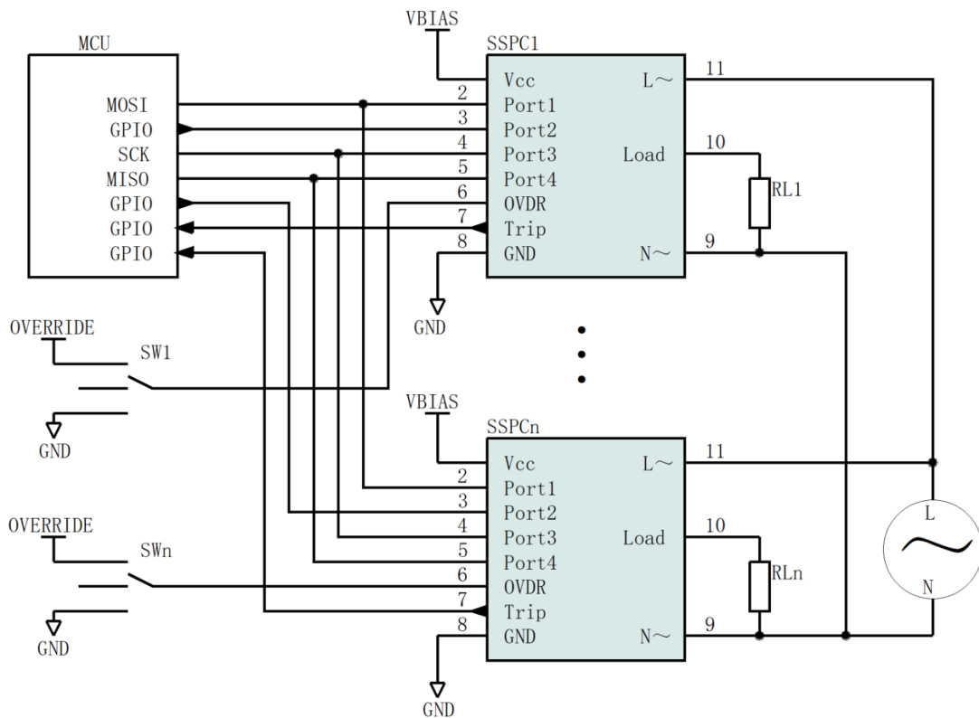
图7 多 SPI 接口模块互联
