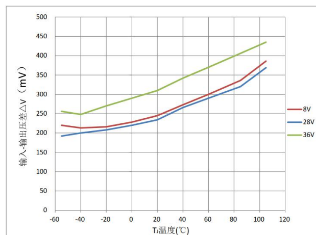
图6 输入-输出压差 \Delta V 与温度特性
