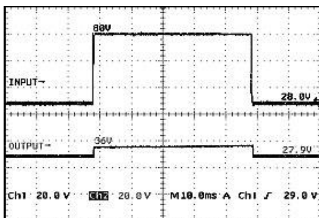
图3 过压浪涌输入输出波形
