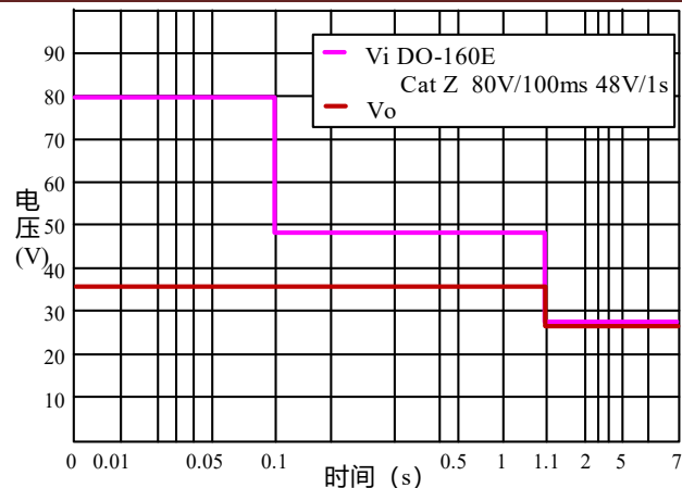
图 8 典型输出特性
