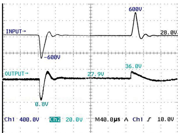
图5 尖峰脉冲输入-输出波形
