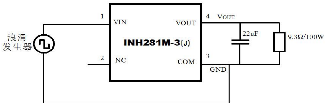
图2 INH281M-3 测试电路图
