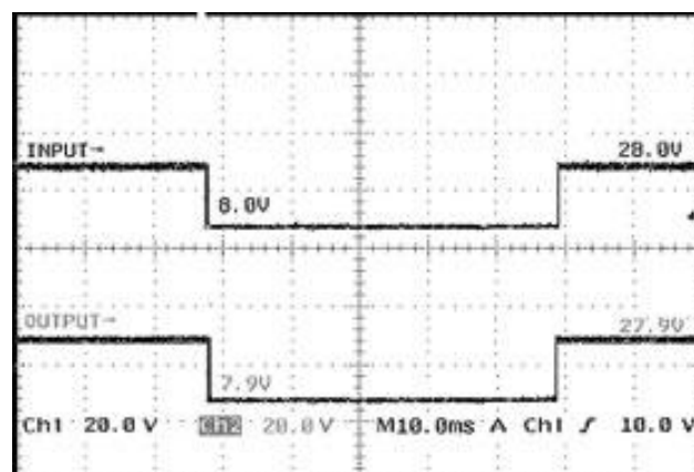
图4 欠压浪涌输入输出波形
