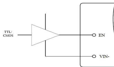
图10 逻辑电平抑制电路
