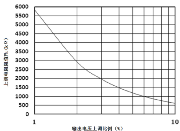
图11 上调电阻阻值 vs.电压上调比例
