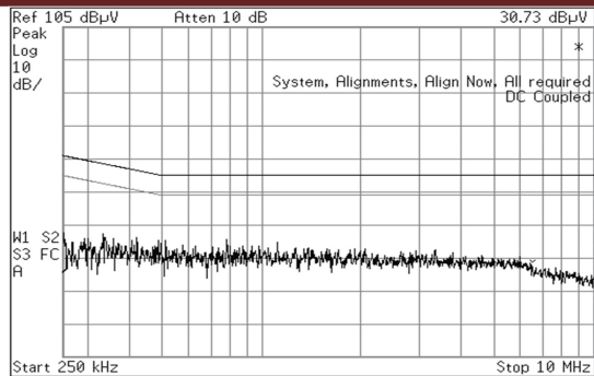
图7 电磁传导发射特性 (前置 MFS 滤波器)
