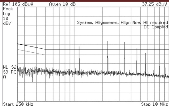
图6 电磁传导发射特性 (未接滤波器)
