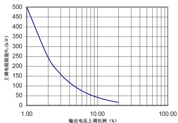
图12 下调电阻阻值 vs.电压下调比例
