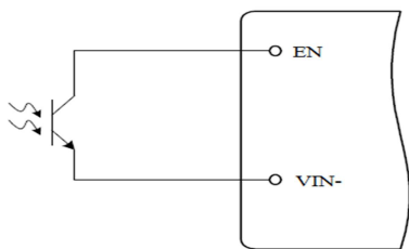
图8 光耦抑制电路
