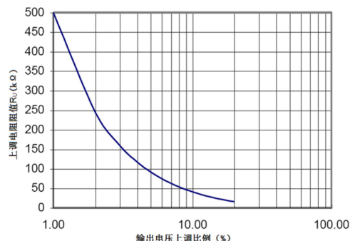
图12 下调电阻阻值 vs. 电压下调比例
