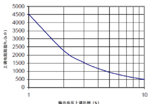
图11 上调电阻阻值 vs. 电压上调比例
